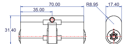
Union Double (Oval)
