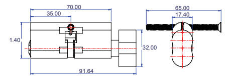
Thumbturn Union (Oval)
