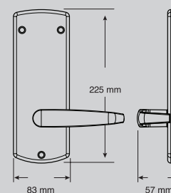
E2000 Interior
