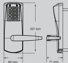
E2000 Exterior
